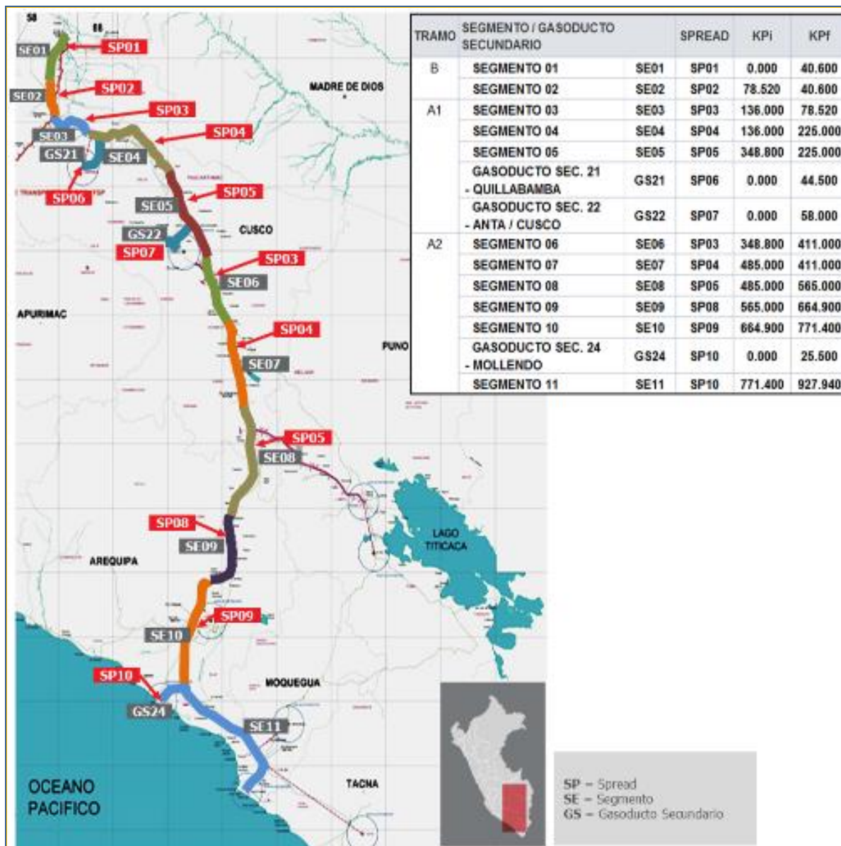
FRENTES DE TRABAJO PARA LA CONSTRUCCIÓN DE LOS DUCTOS
