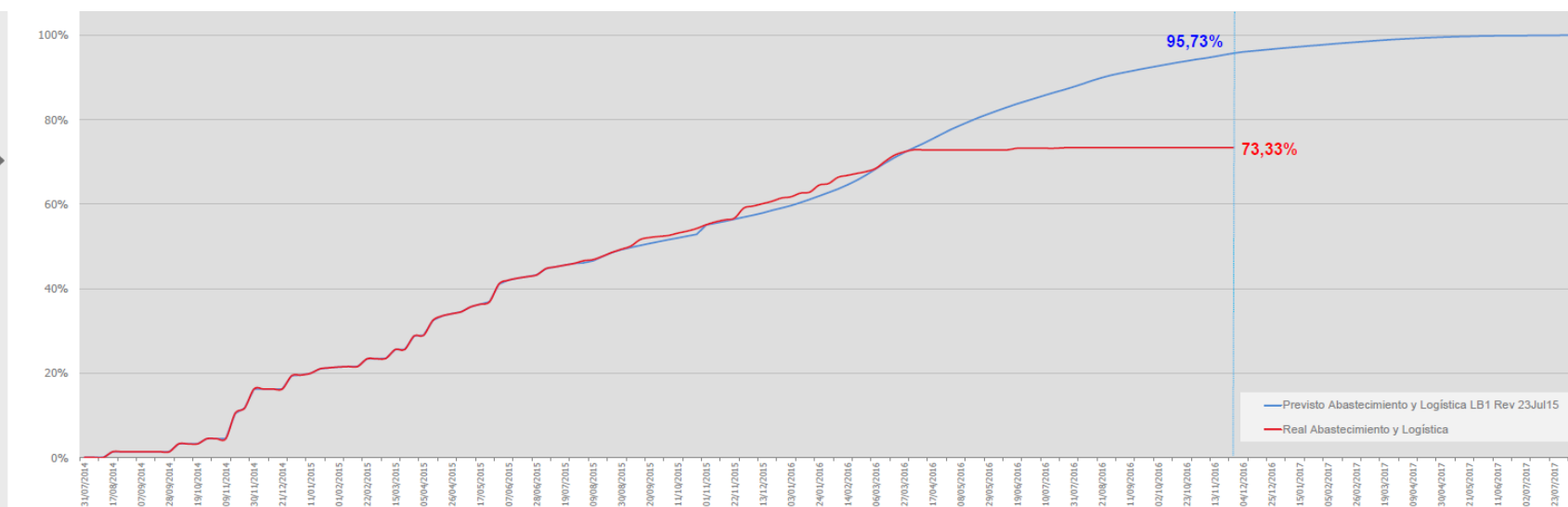
Estado de Avance - Curva de Abastecimiento y Logística, al 27.11.2016
