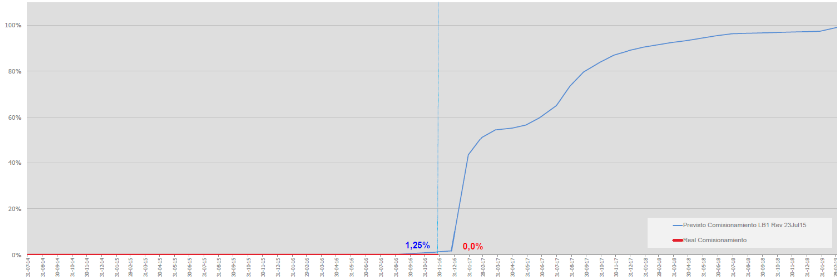
Estado de Avance - Curva de Comisionamiento, al 27.11.2016
