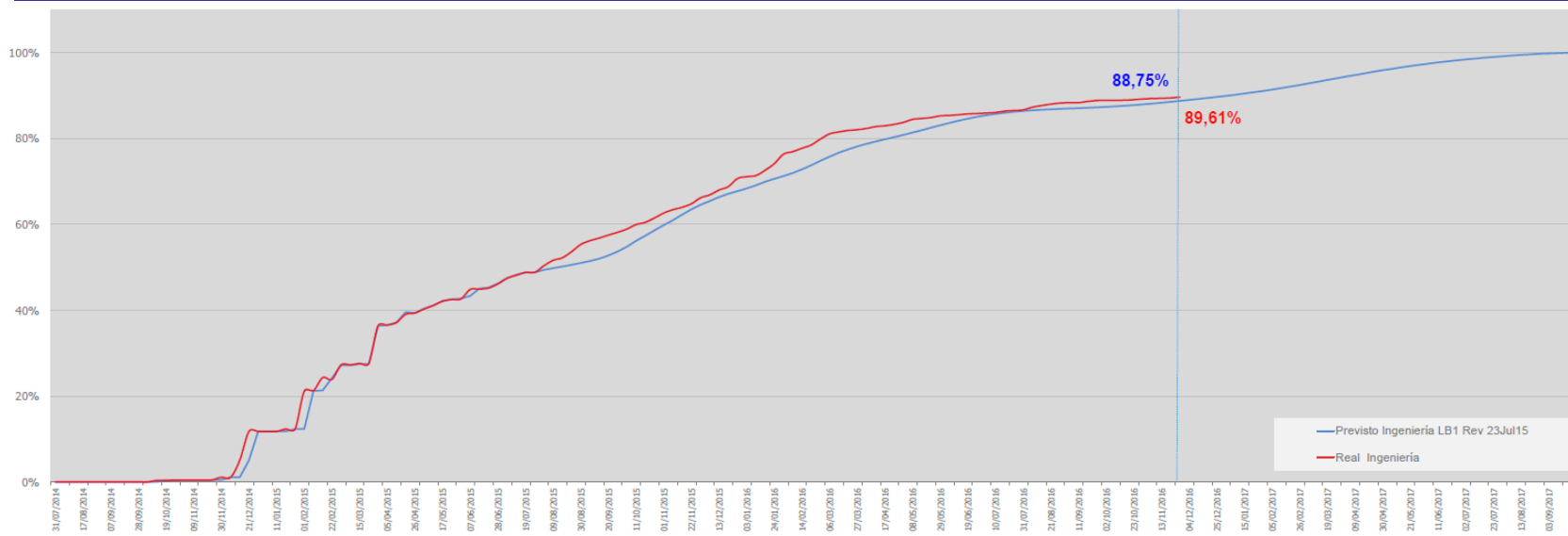
Estado de Avance - Curva de Ingeniería, al 27.11.2016
