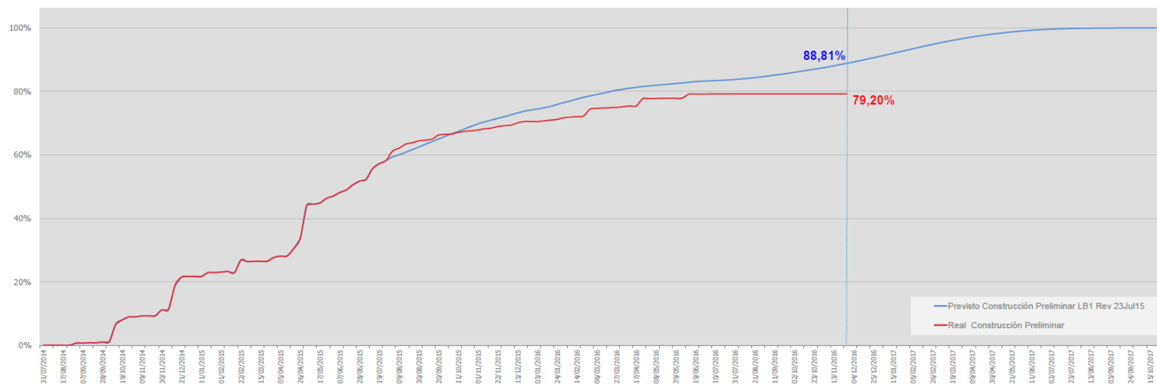
Estado de Avance - Curva de Construcción Preliminar (accesos, acopios, campamentos), al 27.11.2016.
