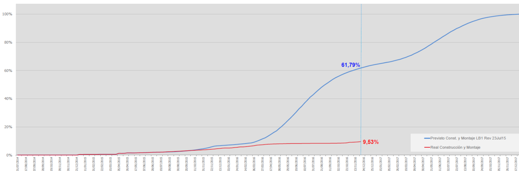
Estado de Avance - Curva de Construcción y Montaje, al 27.11.2016.
