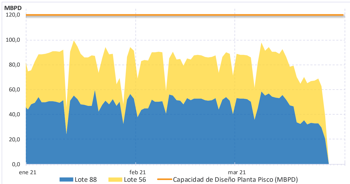
Gráfico 20. Gas Natural Procesado por Lotes y capacidad de Diseño de Planta Pisco (en MBPD) División de Supervisión de Gas Natural [Reporte Diario de Pluspetrol al OSINERGMIN, 2021]
