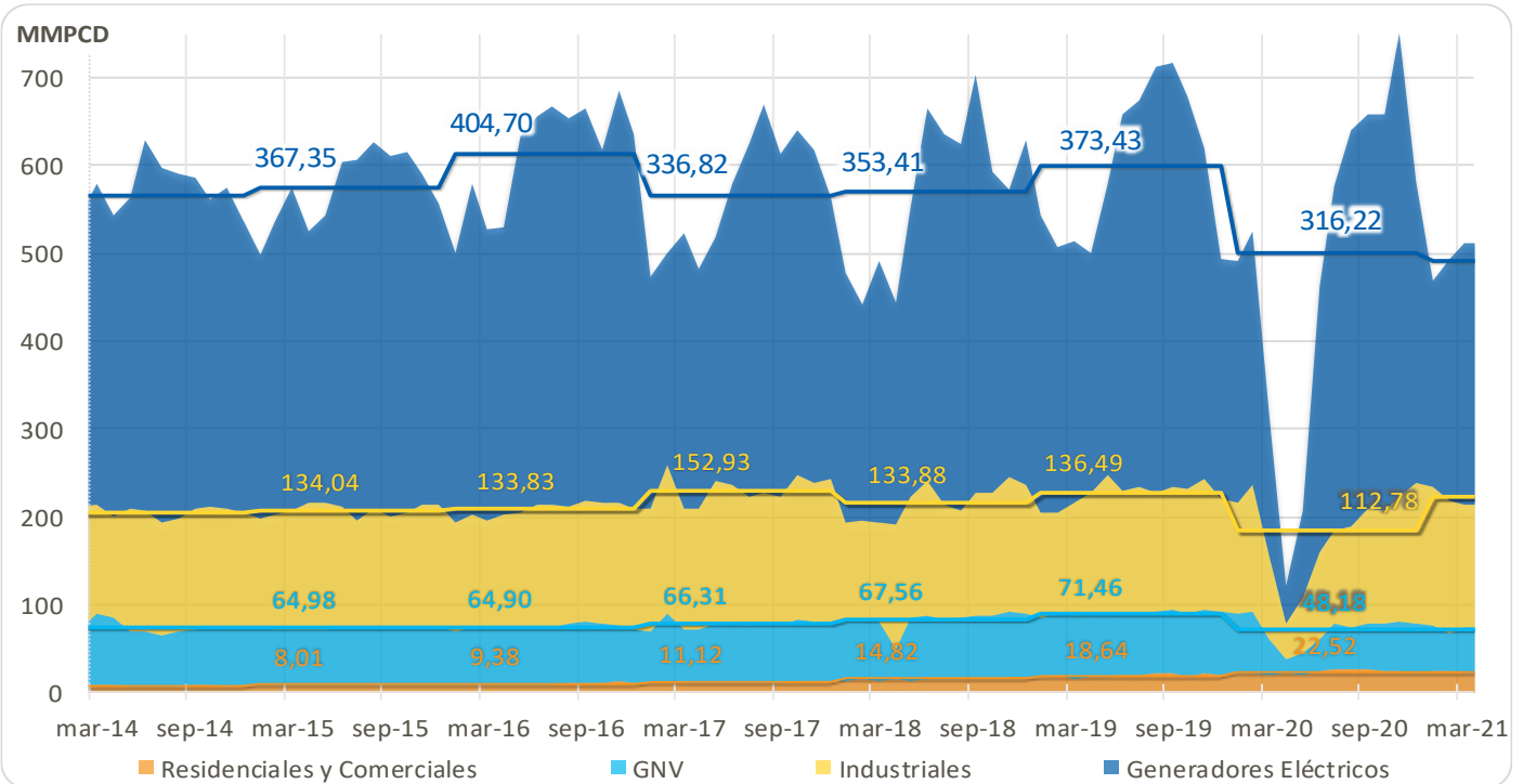
Gráfico 29. Consumo Promedio Mensual del Mercado Interno de Gas Natural de Camisea – 2021 (en MMPCD) División de Supervisión de Gas Natural [Elaboración Propia]
