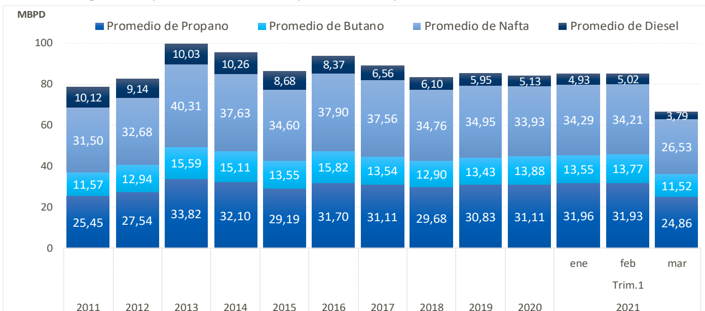
Gráfico 21. Productos Finales Obtenidos del Procesamiento de Líquidos de Gas Natural (en MBPD) División de Supervisión de Gas Natural [Reporte Diario de Pluspetrol al OSINERGMIN, 2021]
