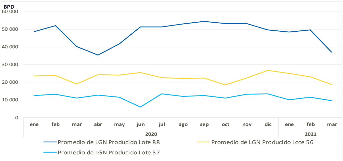
Gráfico 13. Producción Promedio Mensual de Líquidos de Gas Natural, Principales Lotes (en MMPCD) División de Supervisión de Gas Natural [Reporte Diario de Pluspetrol al OSINERGMIN, 2021]
