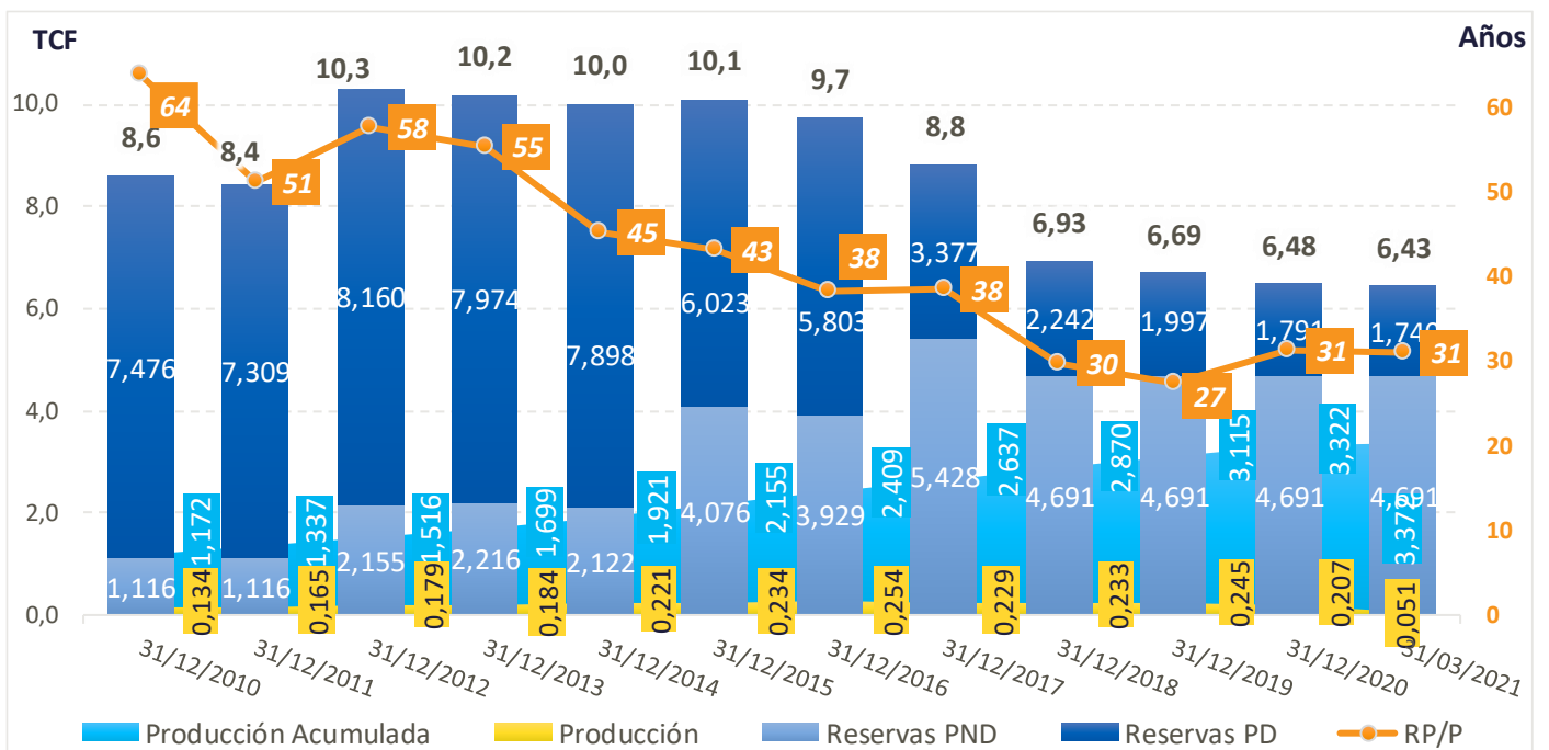
Gráfico 40. Reservas y Producción Acumulada. Lote 88 (en TCF) División de Supervisión de Gas Natural [Libro Anual de Recursos de Hidrocarburos 2018, Minem]
