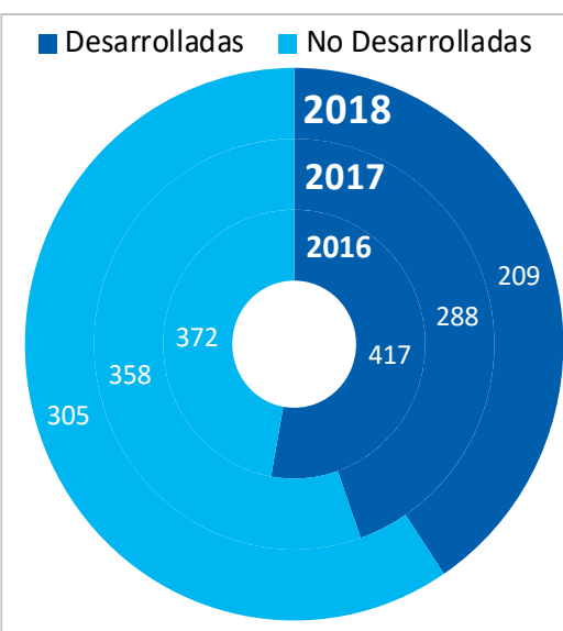
Gráfico 9. Reservas Probadas de Líquidos de Gas Natural al 31 de diciembre de 2018 (en MMSTB [10 6 ])
