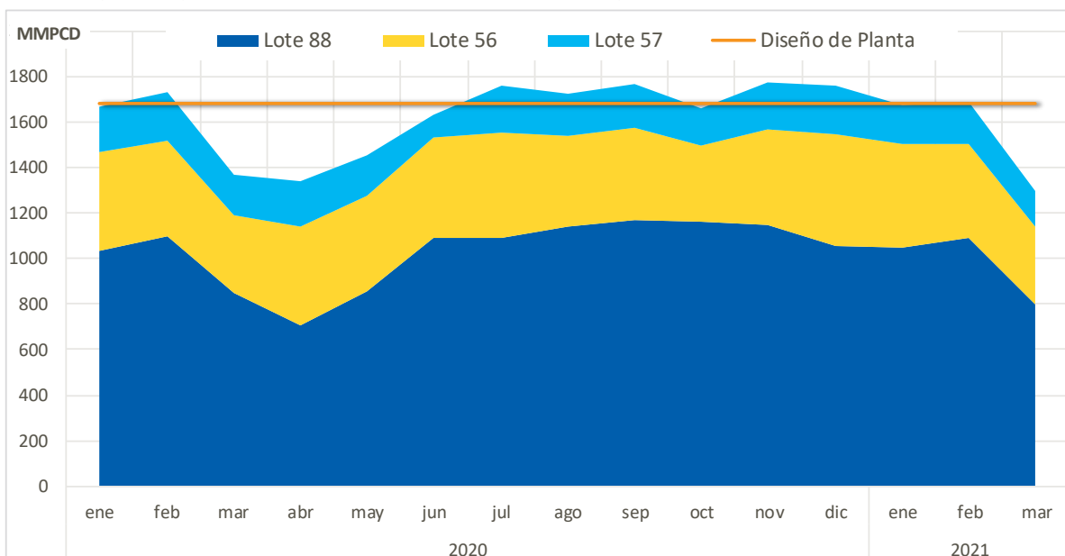
Gráfico 19. Gas Natural Procesado por Lotes y capacidad de Diseño de Planta (en MMPCD)
