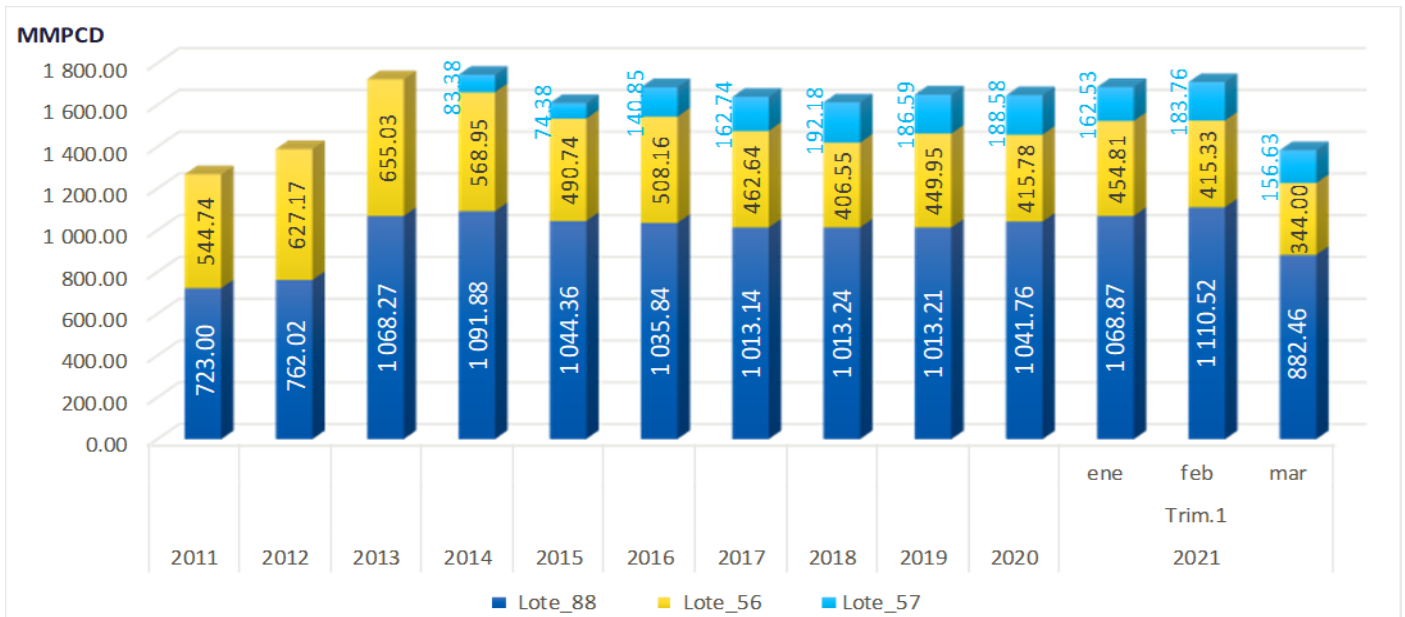
Gráfico 11. Producción Promedio Mensual de Gas Natural Húmedo al 2020, Principales Lotes (en MMPCD) División de Supervisión de Gas Natural [Reporte Diario de Pluspetrol al OSINERGMIN, 2021]
