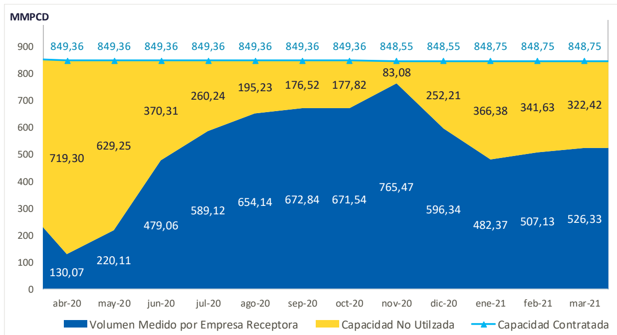
Gráfico 24.. Capacidad de Transporte de Gas Natural no Utilizada en el Mercado Interno (en MMPCD) División de Supervisión de Gas Natural [Facturas TgP reportadas al OSINERGMIN, 2021]
