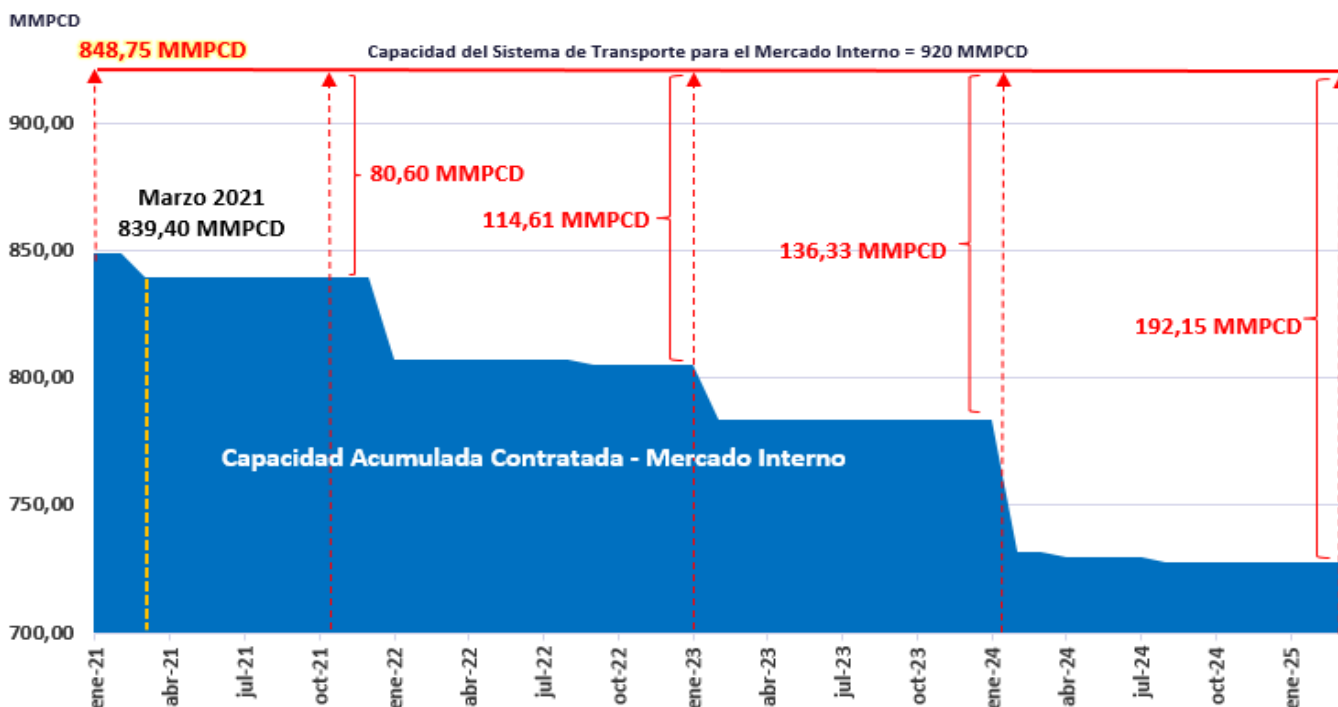
Gráfico 53. Demanda Comprometida de Transporte de Gas Natural hasta la 22da Oferta Pública División de Supervisión de Gas Natural
