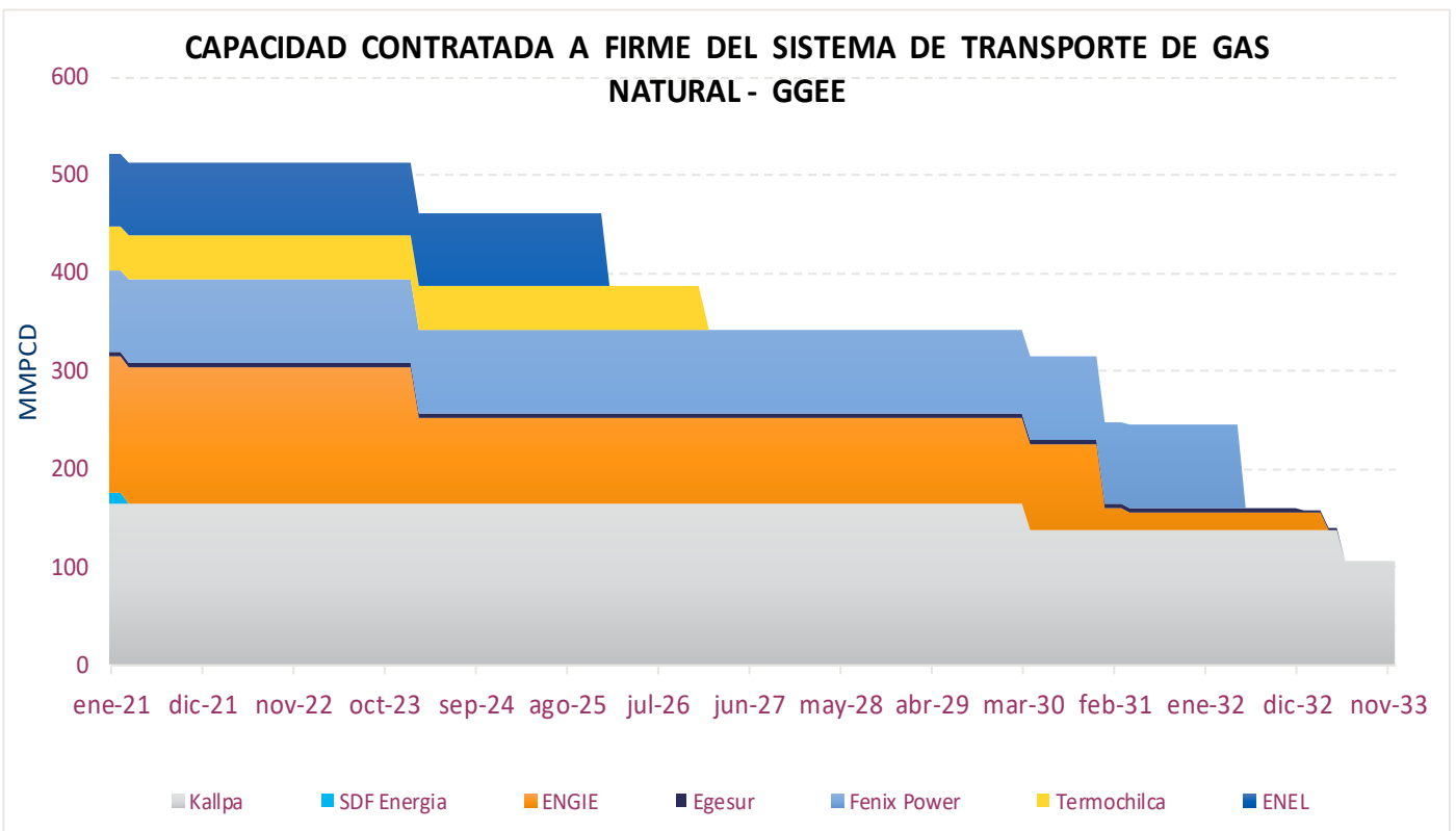
Gráfico 50. Capacidad Contratada de Transporte de Gas. Generadores Eléctricos (en MMPCD) División de Supervisión de Gas Natural
