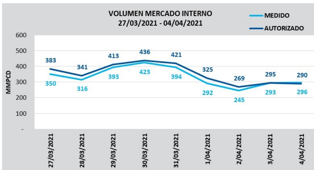
Gráfico 54. Volúmenes Autorizados y Medidos durante el periodo de Mecanismo de Racionamiento activado por RD 160-2020-MINEM/DGH División de Supervisión de Gas Natural
