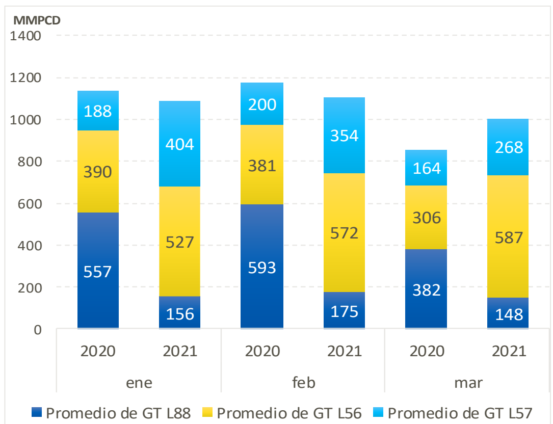
Gráfico 23.. Comparación de Gas Natural Transportado por Lotes T1-2020 vs T1-2021 (en MMPCD) División de Supervisión de Gas Natural [Reporte Diario de TgP, OSINERGMIN, 2021]
