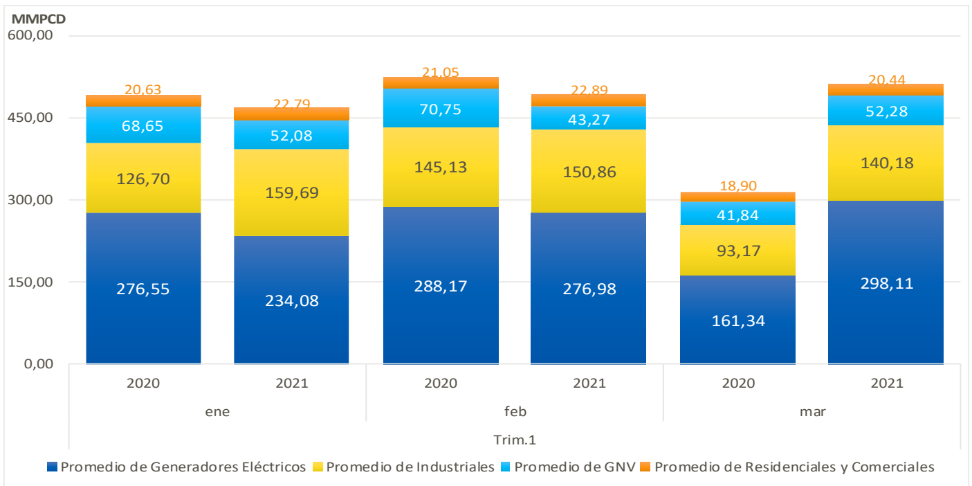
Gráfico 31. Consumo Promedio Mensual del Mercado Interno de Gas Natural de Camisea – marzo 2021 (en MMPCD) División de Supervisión de Gas Natural [Elaboración Propia]
