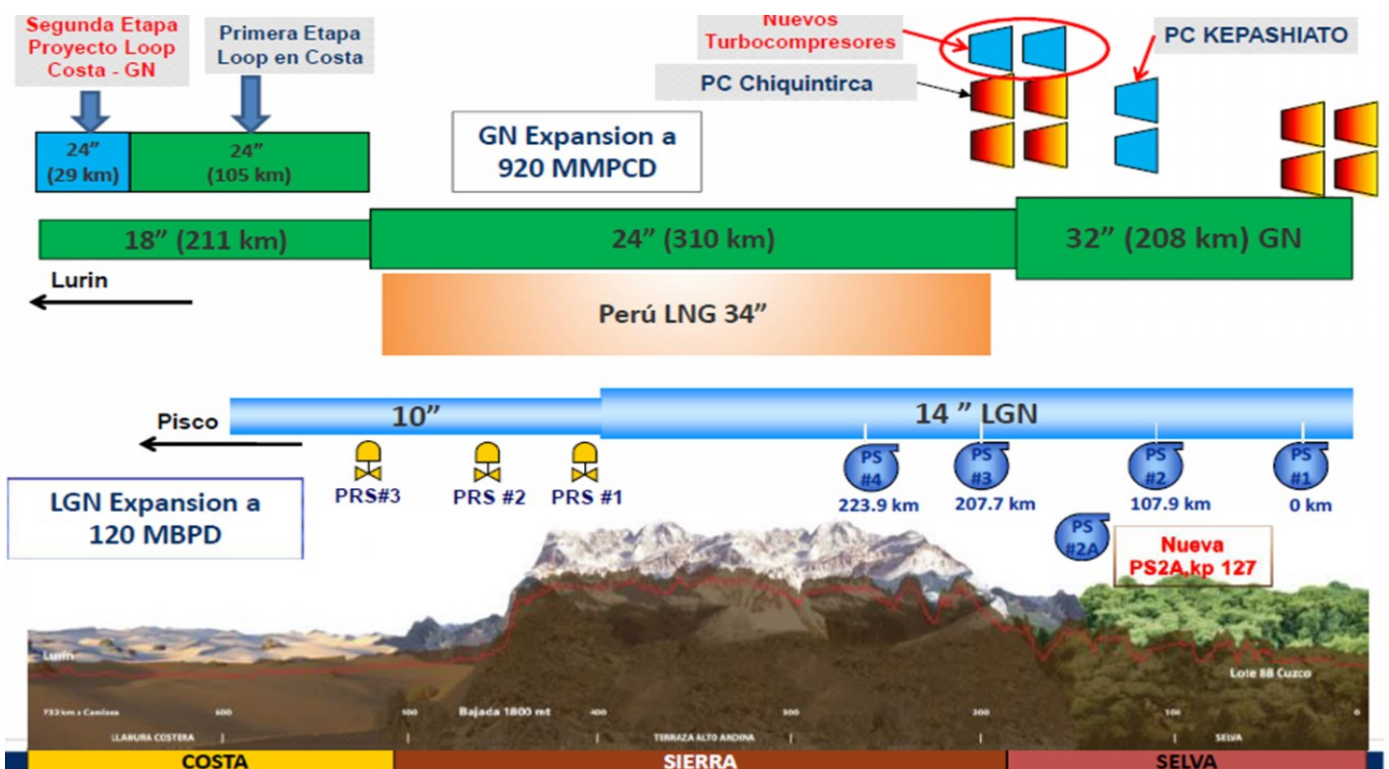
Ilustración 4. Capacidad de Transporte de Gas Natural y Líquidos de Gas Natural desde Camisea a la Costa, Ducto Perú LNG -
