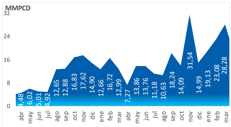
Gráfico 26. Volumen Transferido Entre Empresas Receptoras (en MMPCD) División de Supervisión de Gas Natural [Facturas TgP reportadas al OSINERGMIN, 2021]
