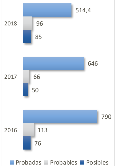
Gráfico 10. Reservas de Líquidos de Gas Natural al 31 de diciembre de 2018 (en MMSTB [10 6 ]) [DGH-MINEM Libro Anual de Recursos de Hidrocarburos, 2018]
