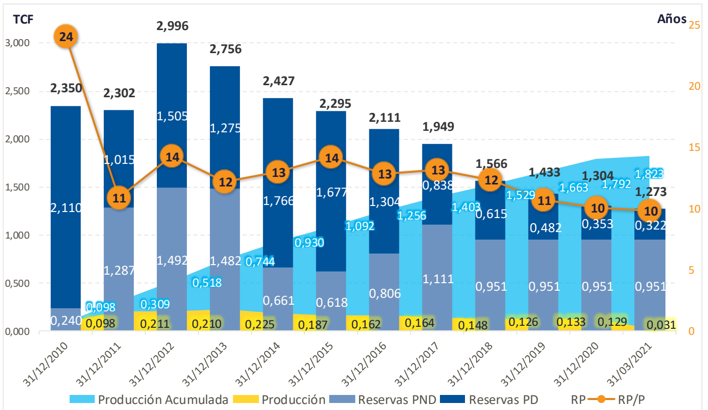
Gráfico 39. Reservas y Producción Acumulada. Lote 56 (en TCF) División de Supervisión de Gas Natural [Libro Anual de Recursos de Hidrocarburos 2018, Minem]
