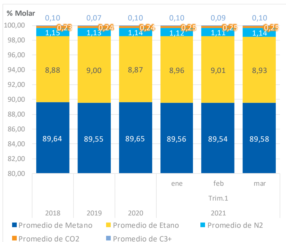
Gráfico 25. Composición Porcentual del Gas Natural Transportado en el City Gate Lurín (en MMPCD) División de Supervisión de Gas Natural [Certificados de Entrega TgP Reportadas al OSINERGMIN, 2021]
