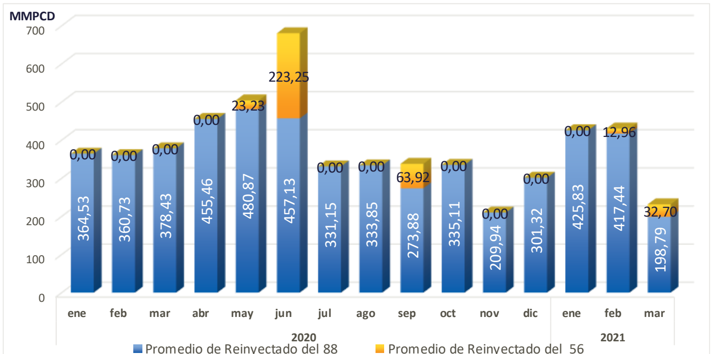
Gráfico 18. Reinyección de Gas Natural, por Lotes (en MMPCD)
