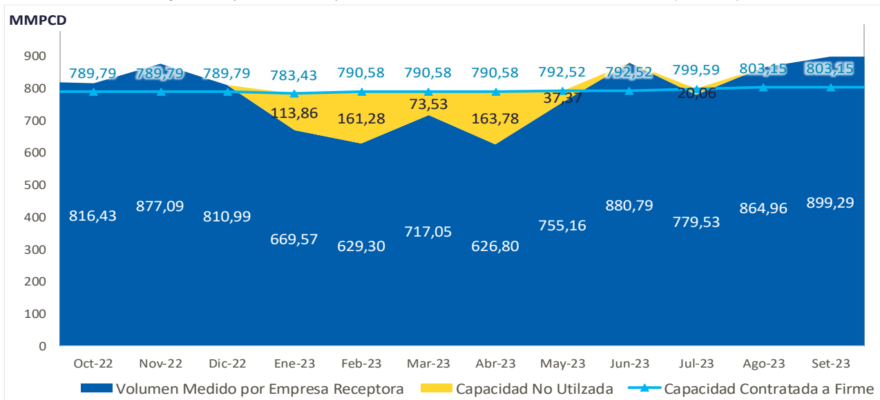
Gráfico 26. Capacidad de Transporte de Gas Natural no Utilizada en el Mercado Interno (en MMPCD)
