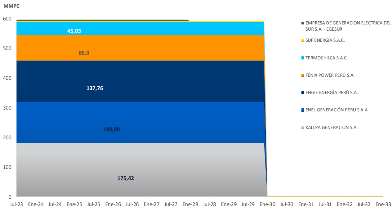
Gráfico 50. Volumen Contratado de Suministro para GGEE. Pluspetrol (en MMPCD)
