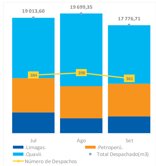
Gráfico 38 Total Despachado Mensual Volumen de Gas Natural Licuefactado al T3-2023 (en m 3 )
