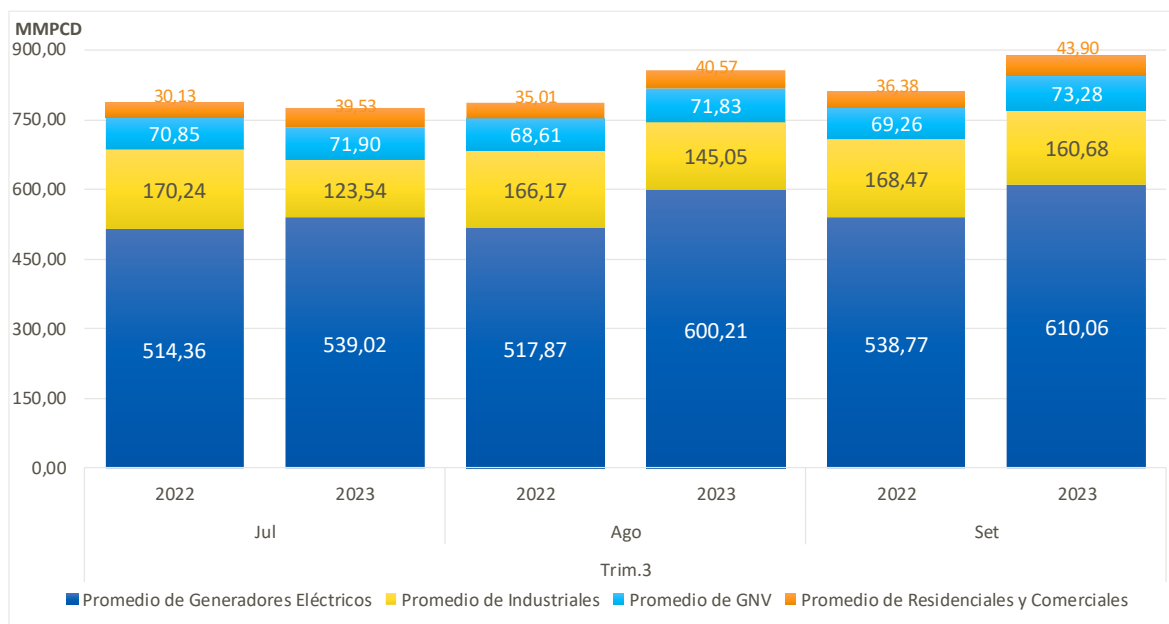
Gráfico 33. Consumo Promedio Mensual del Mercado Interno de Gas Natural de Camisea – T3-2022 vs T3-2023 (en MMPCD)
