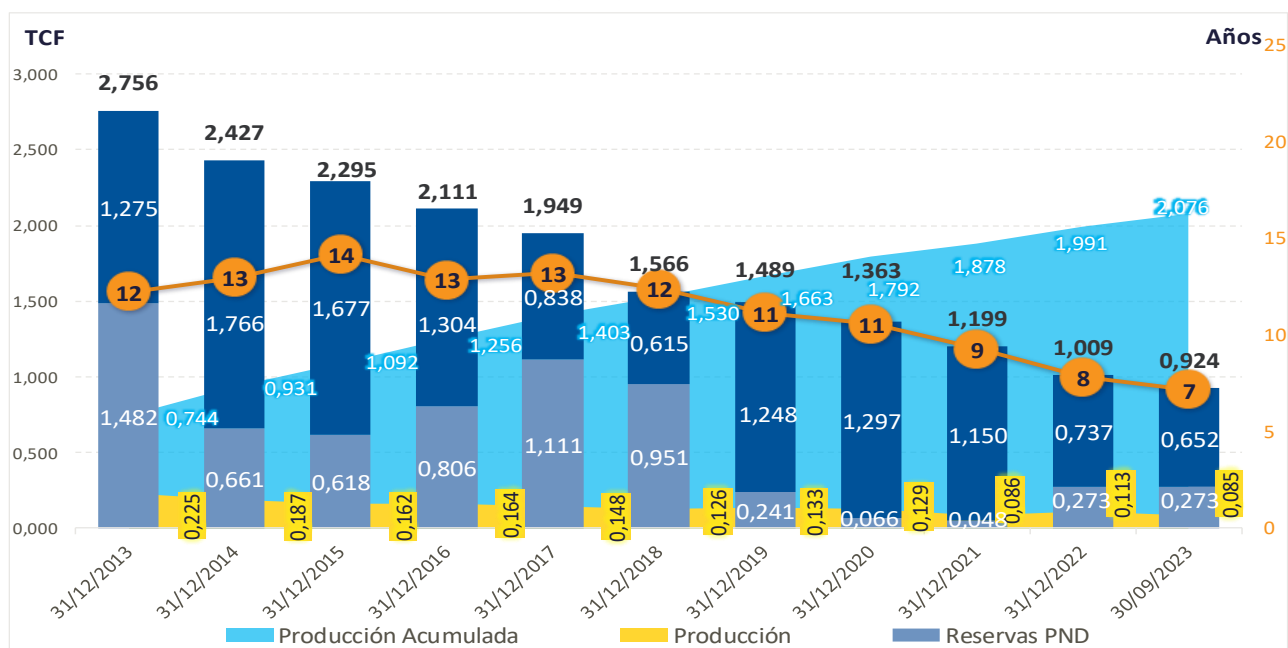
Gráfico 40. Reservas y Producción Acumulada. Lote 56 (en TCF)
