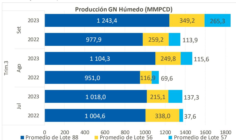
Gráfico 14. Comparación de Producción Promedio Mensual de Gas Natural Húmedo del Primer
