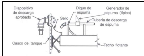
Gráfico 7.- Modelo de aplicación de espuma en superficie en tanque de techo flotante.
