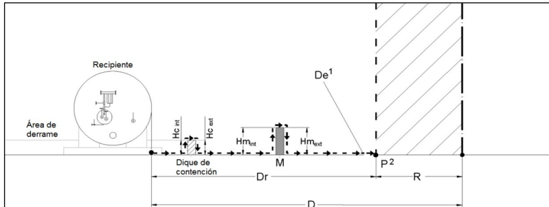
Figura A.3 - Distancia de seguridad. Metodología de medición. Reducción de la distancia. Consideración de la altura del muro reductor
