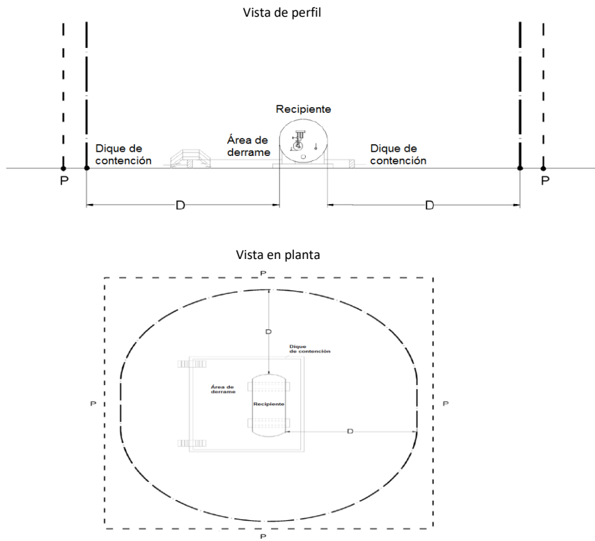
Figura A.1 - Distancia de seguridad. Metodología de medición.
