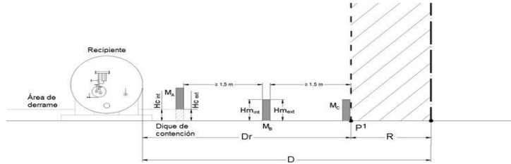
Figura A.4 - Distancia de seguridad. Metodología de medición. Reducción de la distancia. Alternativas de aplicación del muro reductor (elementos lineales)
