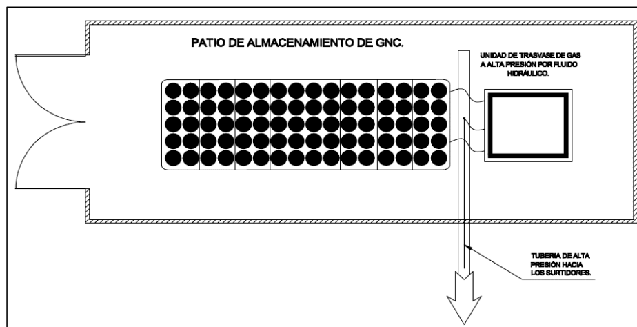
Figura 3 - Traslado del GNC por medio de un fluido hidráulico
