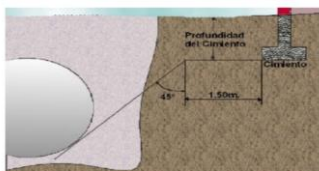
FIGURA 1 - Distancia de tanque de combustible líquido enterrado
