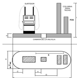
FIGURA 3 - Dimensiones de las islas de los dispensadores
