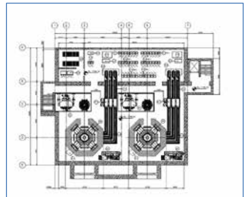
Vista de planta del equipamiento
